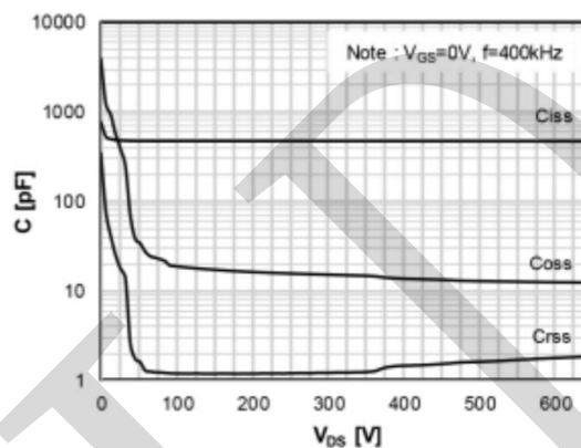
Fig. 2 Capacitances
